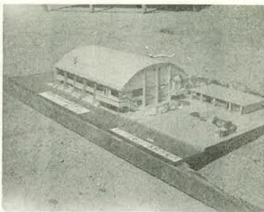
安富祖小中学校体育館完成後の 模型写真正面
