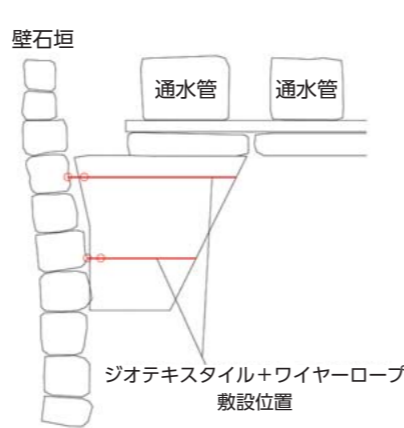
図2 ジオテキスタイル計画図（橋内部の断面図）
