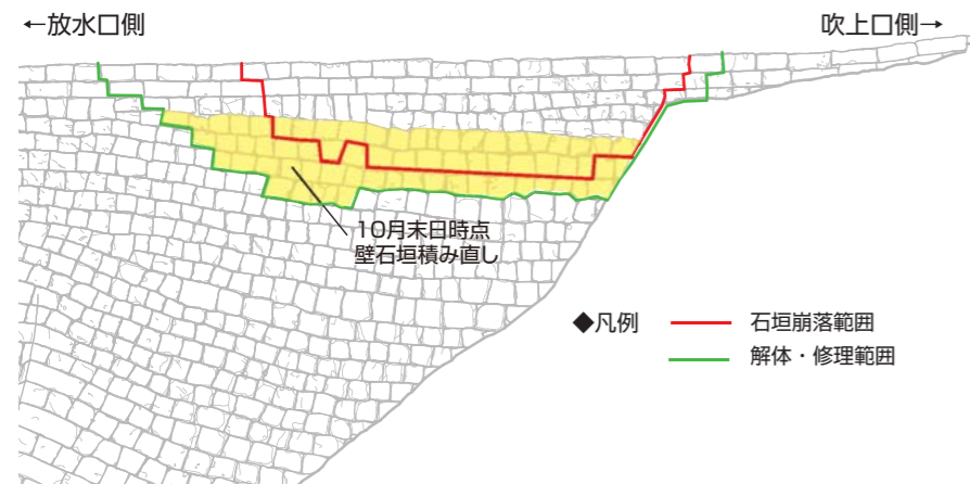
図1 石垣の修理範囲（立面図）
