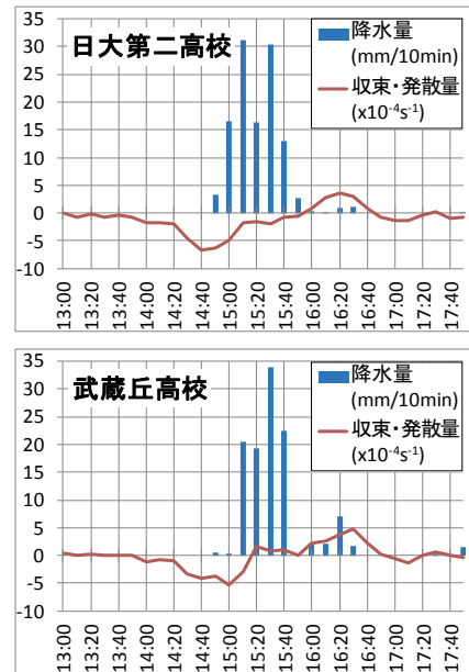
図5 日大第二高校（上）、武蔵丘高校（下）における2011年8月26日の10分間降水量と収束・発散量の時間変化（収束・発散量は、各観測点周囲の4格子点における平均値）
