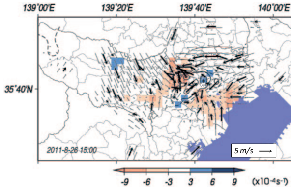
図4 2011年8月26日15時00分の収束・発散量分布（各観測点の風を約3 km 間隔に格子点化した風（細矢印）から算出、等値線は図3と同じ）
