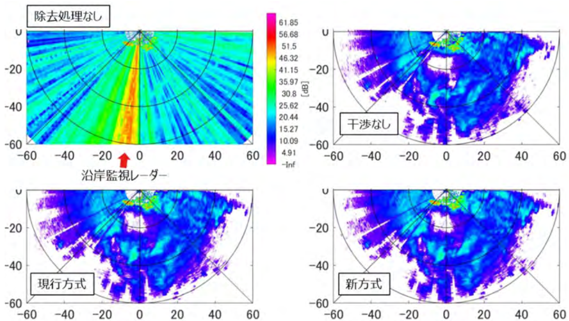
図 2. 2-17 干渉除去によるPPI (電力、固体素子型パルス条件4、仰角1.4deg.)
