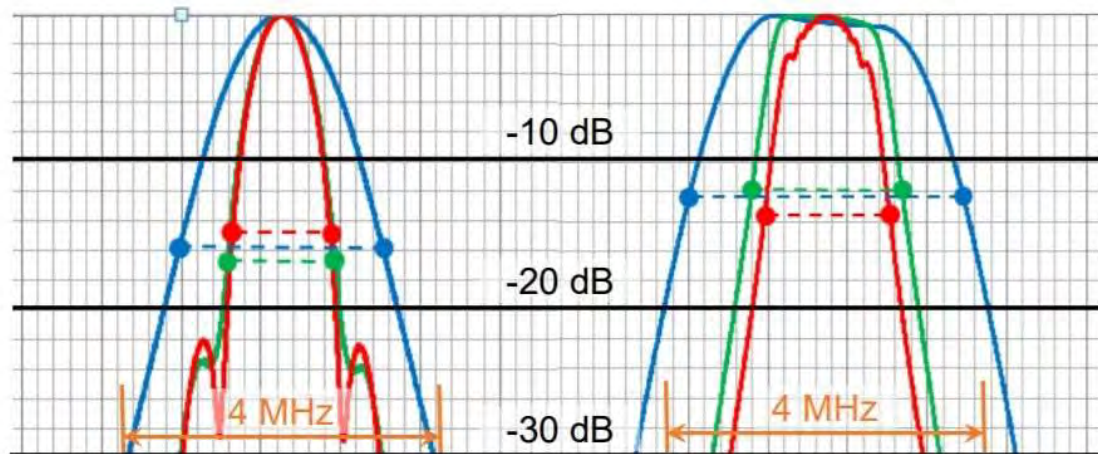
図 2. 4 4 - 4 OBW の測定方法の根拠
