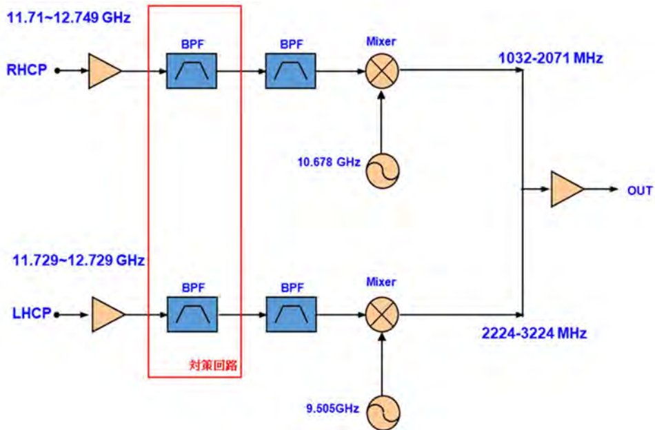
図 4. 2 - 2 ② B P F 追加による対策モデル
