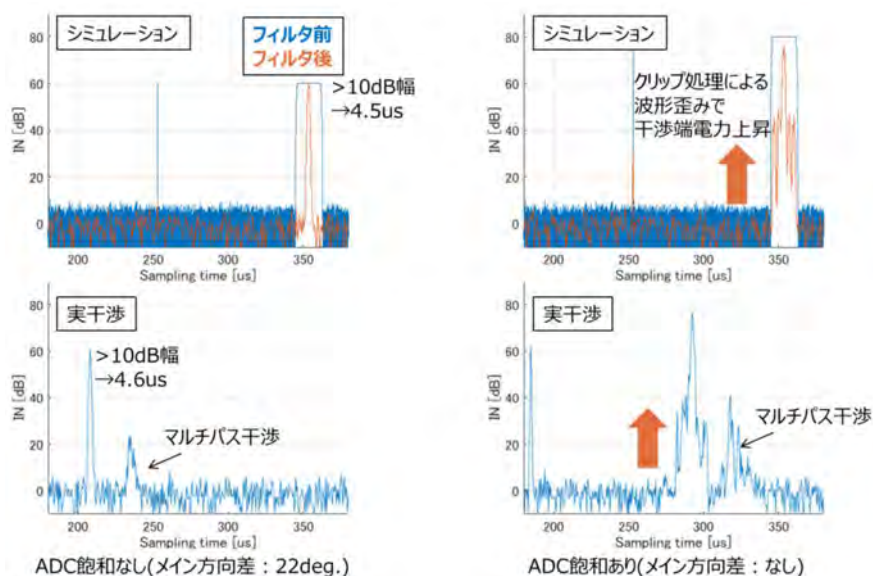
図 2. 2-13 干渉波形
