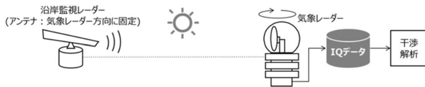
図 2. 2-2. 211 晴天試験概要
