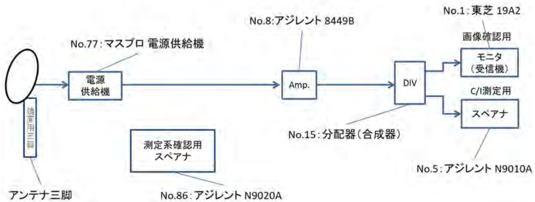
図4. 3-20 干渉試験によるBS受信画像測定系統
