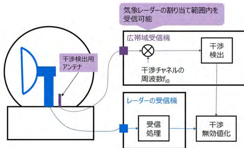
図 2. 1-12 広帯域受信機のシステム概念図
