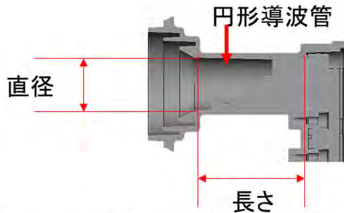
図4. 2-3 ③一次放射器の円形導波管の設計変更による対策モデル
