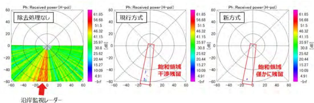
図 2. 2-2. 2-14 干渉除去による PPI (電力、固体素子型パルス条件 4)
