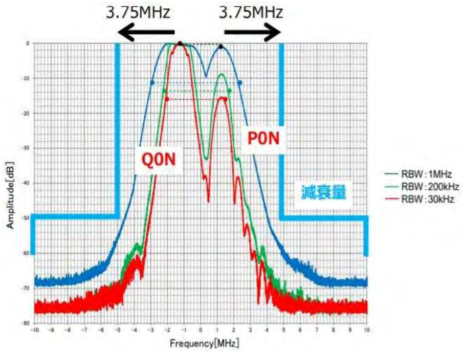
図 2. 4 4 - 3 周波数オフセットについて
