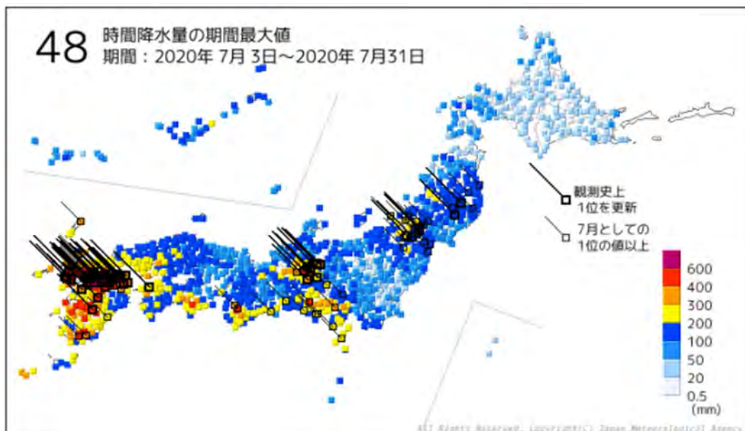
図 1. 1-3 48 時間降水量の期間最大値の分布図 (7 月 3 日～7 月 31 日)
