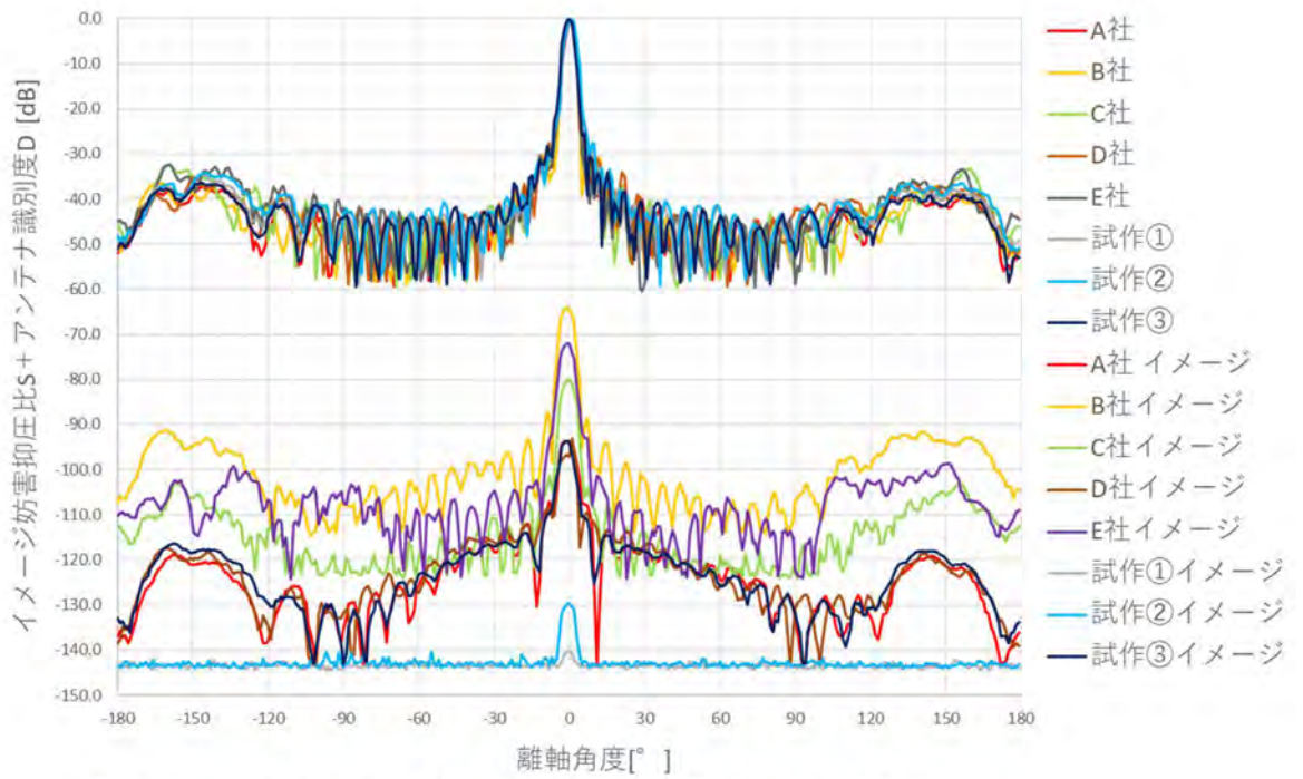
図 4. 3 - 1 1 仰角ポアサイトの水平面パターン (BS-23ch)
