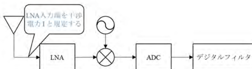
図 2. 22-3 干渉電力 I の規定点
