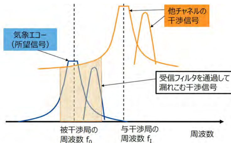
図 2. 1-11 他チャンネルの気象レーダー間干渉時の周波数スペクトル配置
