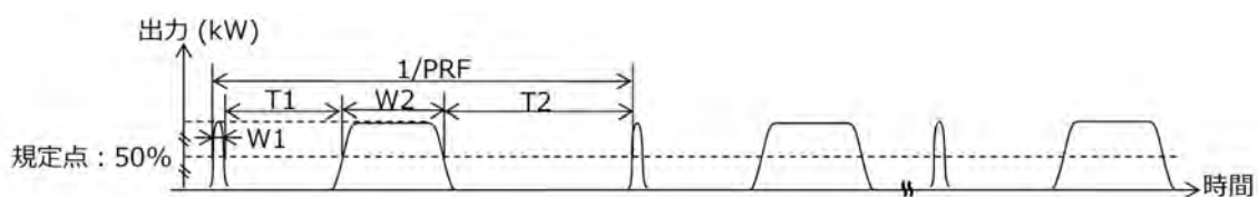
図 5. 2-2 DFS が検出するパルスパターン
