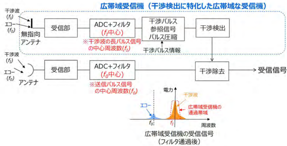
図 2. 1-13 広帯域受信機を用いた干渉検出、干渉除去
