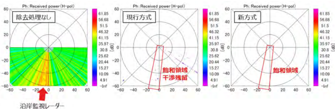
図 2. 2-2. 2-15 干渉除去による PPI (電力、固体素子型パルス条件 7)
