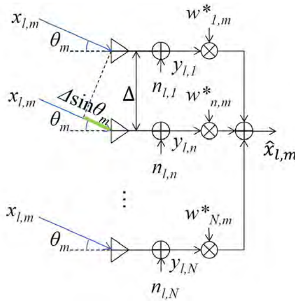
図 2. 1-6 PAWR のシステムモデル
