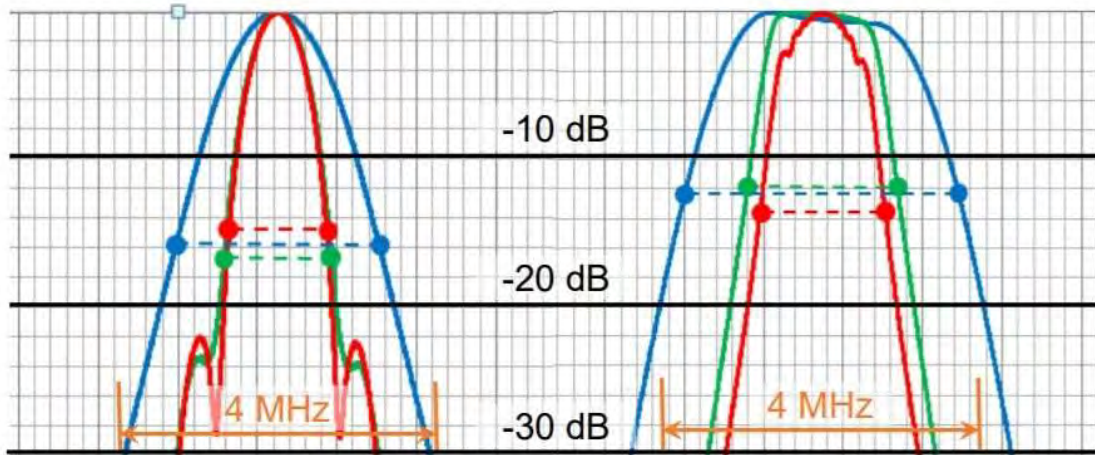
図4 OBWの測定方法の根拠
