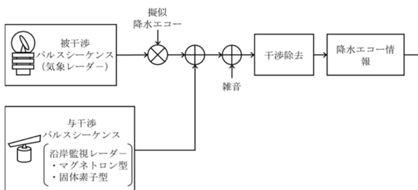
図 2. 22-2 シミュレーション概要
