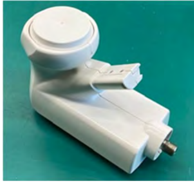
図4. 2-5 ②BPF追加による対策モデル 試作品
