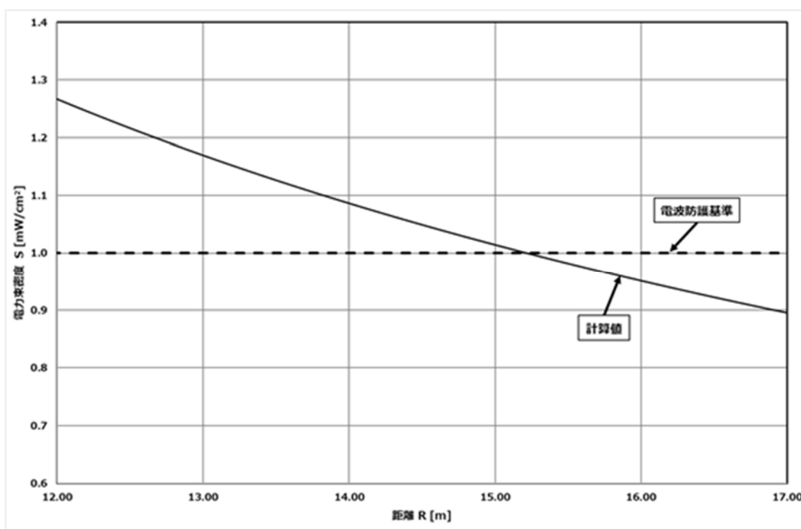
図 2. 4 4 - 2 X 帯高性能型気象レーダーの電波防護指針と適合性 (例)
