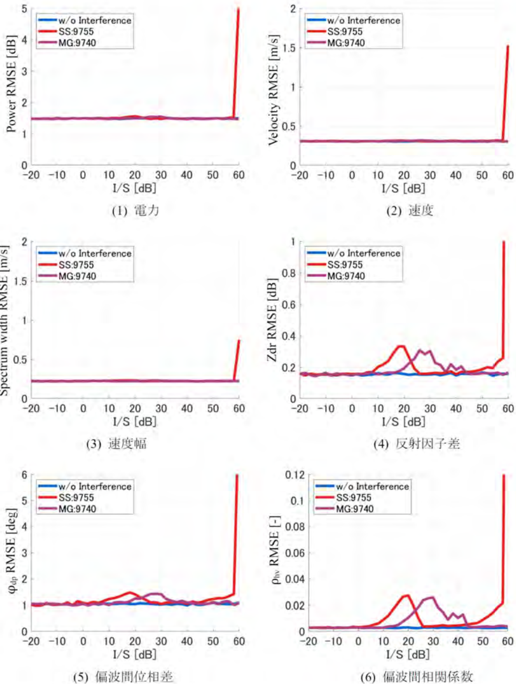
図 2. 2. 2. 2-6 降水エコー推定精度
