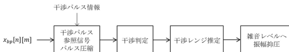
図 2. 1-10 対向レーダー間のパルス情報を利用する干渉低減方式概要図
