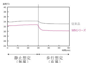
③靴内温度・側面
