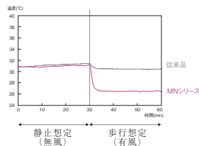
①靴内温度・土踏まず部分
