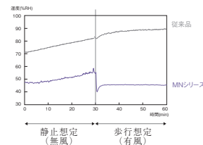
②靴内湿度・土踏まず部分
