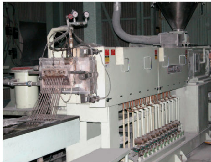
▲ 押出機
