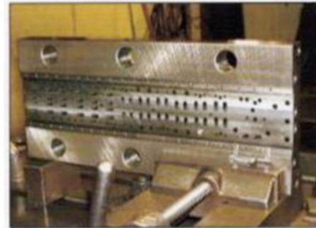
▲ICリードフレーム用スタンピング金型
