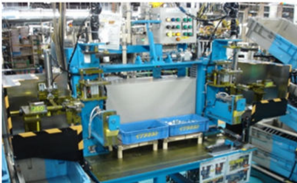
▲組立治具
