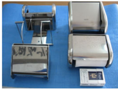
▲ プレス加工
