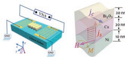
図(2) 表面弾性波を用いたスピン流生成素子の概念図。表面弾性波により強磁性層(Ni)に強磁性共鳴が励起され、スピン流( J_s )が強磁性体層から Cu/Bi_2O_3 界面に注入される。 Cu/Bi_2O_3 界面に到達したスピン流は、逆エデルシュタイン効果により電流( J_c )へと変換され検出される。 参考論文: Hwang et al. PRB (Rapid) (2019)
