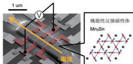
図(1) 収束イオンビーム装置を用いて作製された、『磁気スピンホール効果』測定素子。収束イオンビーム装置を用いることで、新奇物性を示す物質の単結晶を任意の形状に加工することができる。この素子を用いて、スピン蓄積の方向が Mn_3Sn の磁気的な状態に依存する、『磁気スピンホール効果』を初めて実験的に実証した。 参考論文: Kimata et al. Nature,
