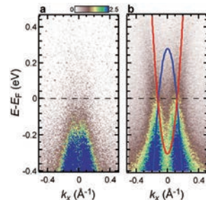
高次高調波レーザー時間分解光電子分光で観測された励起子絶縁体Ta 2 NiSe 5 における光誘起絶縁体-金属転移 a, b はそれぞれ、光励起前、光励起後のスペクトル Photo-induced insulator-to-metal transition in an excitonic insulator Ta 2 NiSe 5 observed by HHG laser TRPES. a, b. Spectra before and after pump, respectively.
