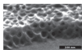
ブロックポリマーのマイクロ相分離構造と超臨界CO 2 処理プロセスを組み合わせ得られるナノ多孔体。高性能反射防止膜や超熱材料への応用が期待される。
