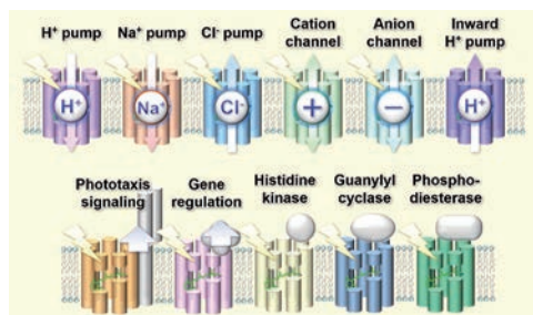
光で多様な機能を発現する微生物型ロドプシン
