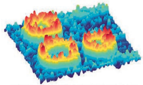
図1: SrTiO 3 基板上のLa 0.6 Sr 0.4 MnO 3 ナノリングの摩擦顕微鏡 (FFM) 像。リングの直径は約100nm、高さは0.4nm。
