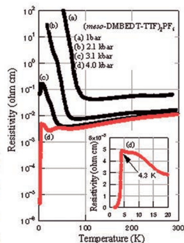
圧力誘起有機超伝導体 \beta -( meso -DMBEDT-TTF) 2 PF 6 のチェッカーボード型電荷秩序と超伝導
