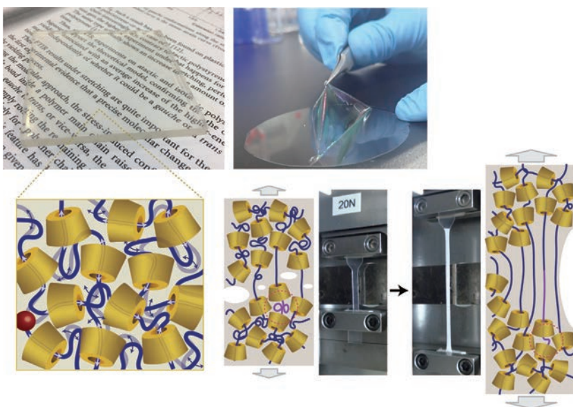
図：環状オリゴ糖を主成分とし、幾何学的に結合した高分子を有する透明プラスチック。ガラス状態にもかかわらず、高分子の鎖は大きく運動しており、これを用いた分離膜への応用が研究されている。高分子鎖と環状オリゴ糖は結合していないため、応力が集中した部分では鎖が環から引き出されることで、堅くても強靱な材料となっている。
