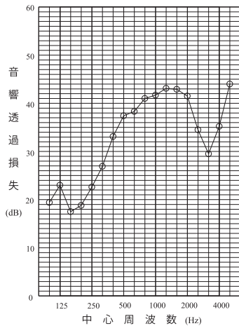
図4 試験結果
