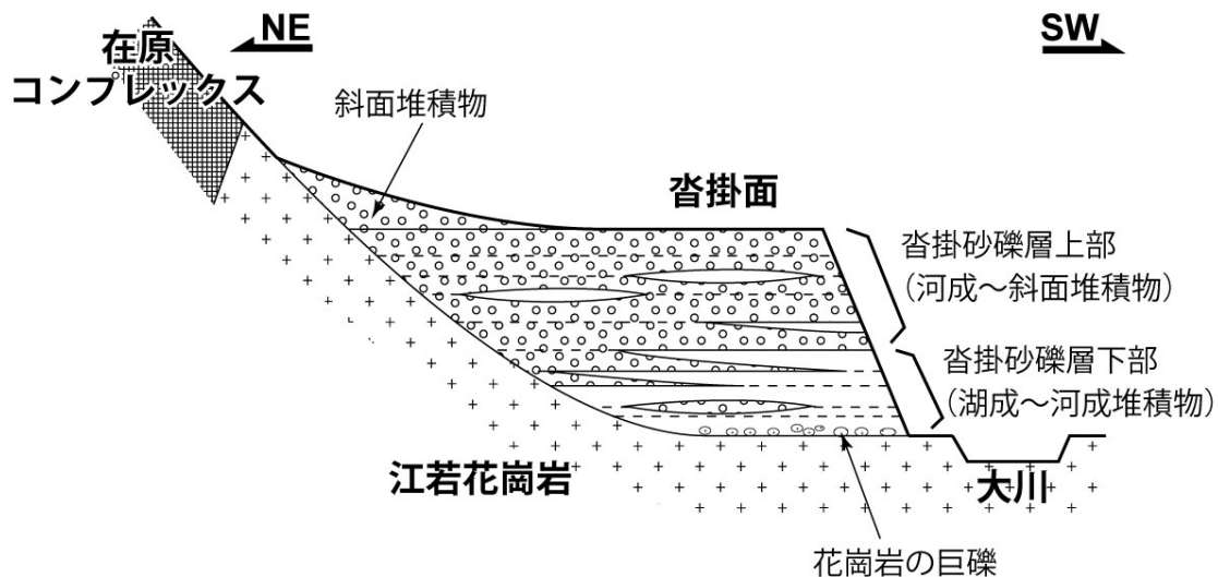
図8 沓掛砂礫層の模式地質断面
