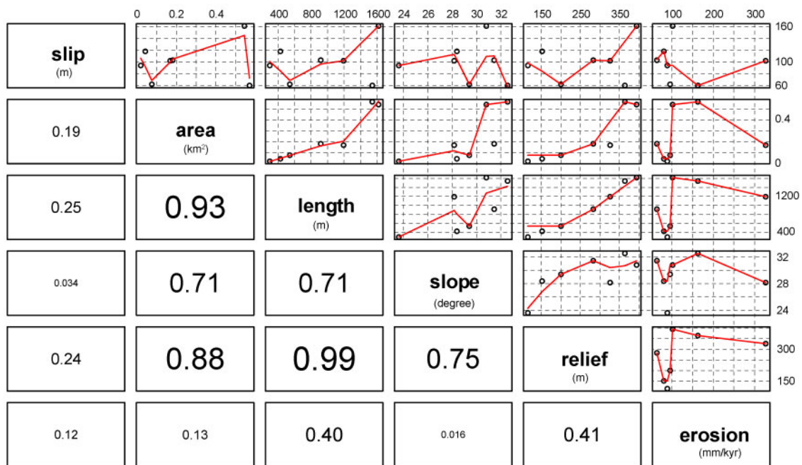
図14 集福寺断層の流域パラメータの散布図行列
