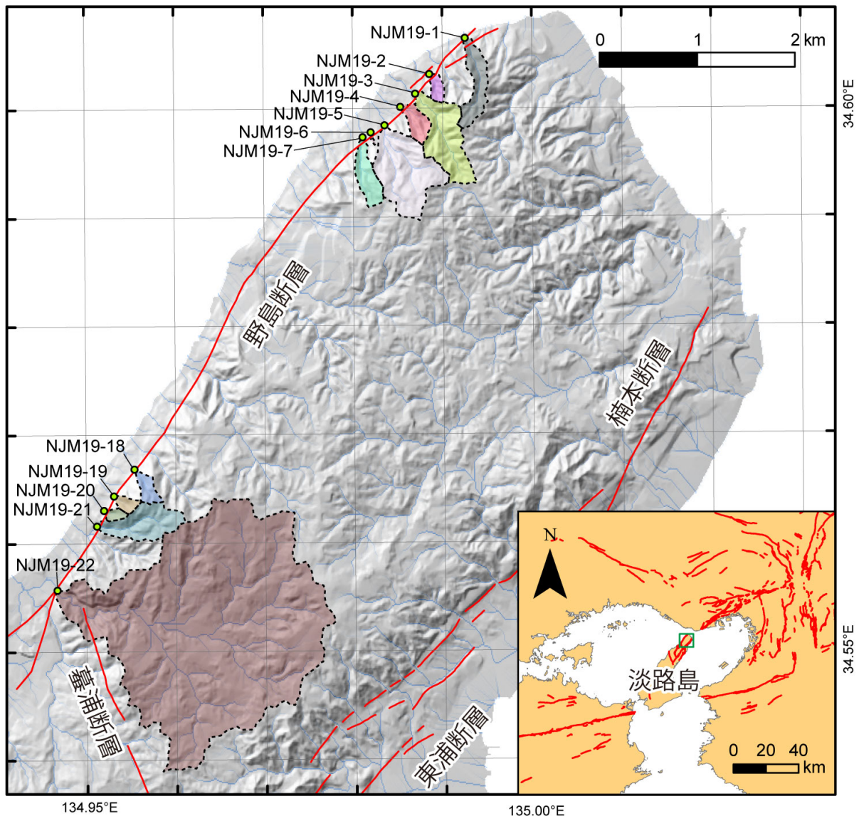
図 13 野島断層沿いの試料採取地点とその流域
