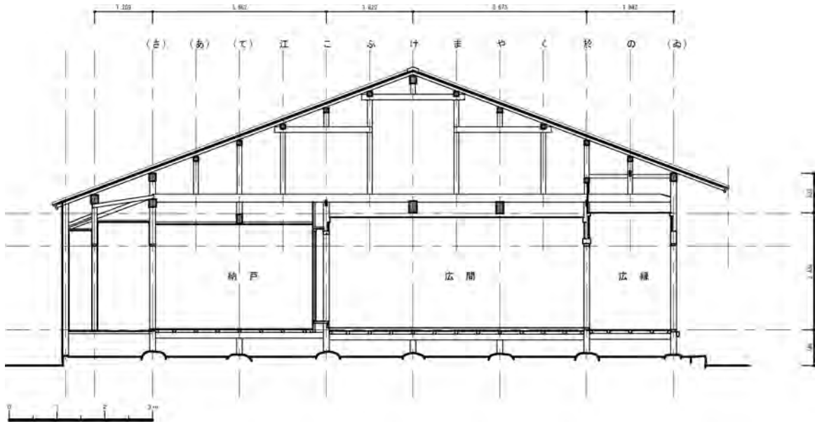
【図3】断面図（七通り）
