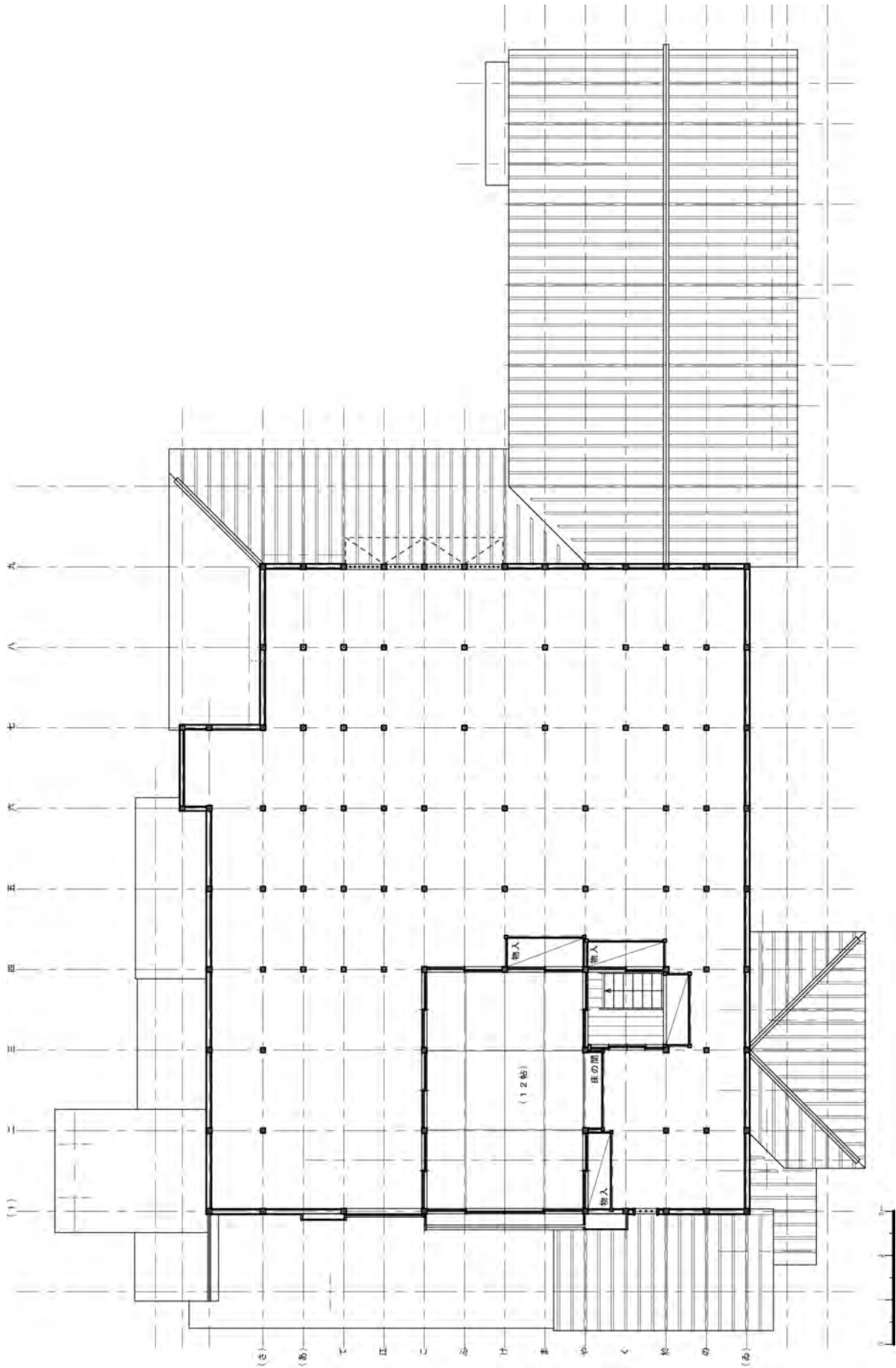
【図2】 2階平面図
