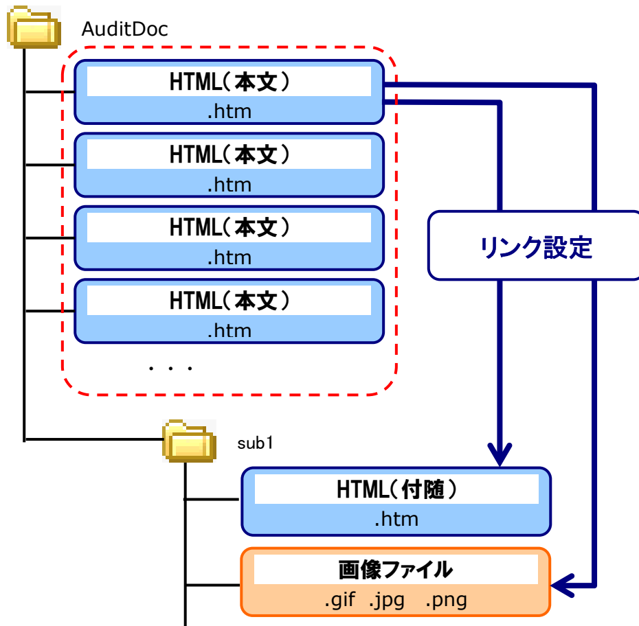
図表 3-7-2 AuditDoc フォルダの構成イメージ
