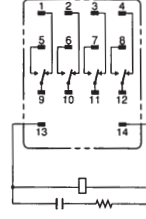
(コイル極性なし)
