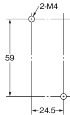
取り付け穴加工寸法
