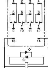
(コイル極性なし)
