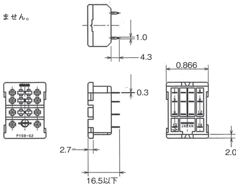
端子配置/内部接続図
