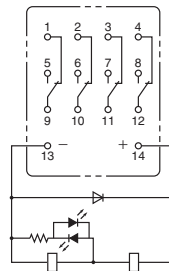
端子配置/内部接続図 (BOTTOM VIEW)
