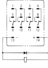
(コイル極性あり)
