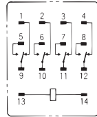
(コイル極性なし)
