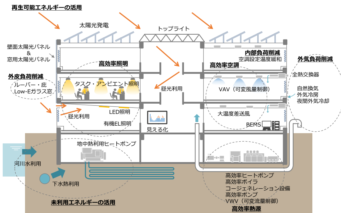
図 4-36 建築物における代表的な措置のイメージ
