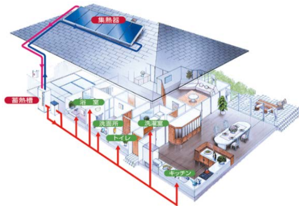
図 4-48 再生可能エネルギー熱の導入：太陽熱
