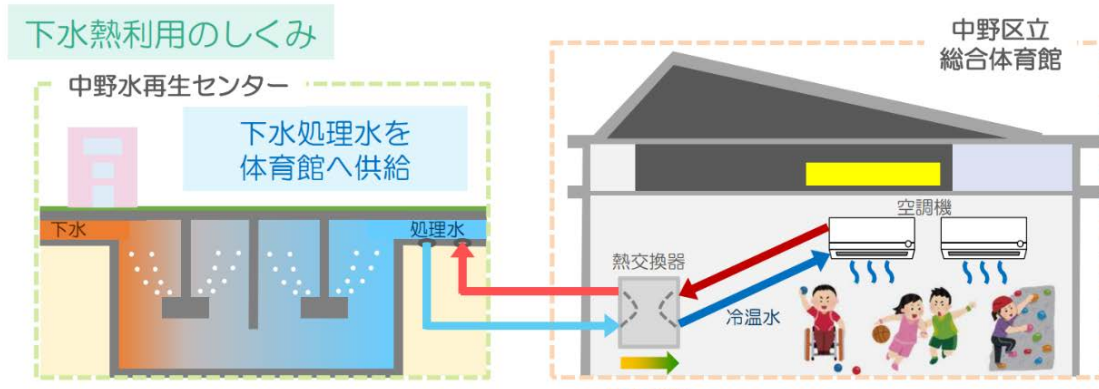
図 4-49 再生可能エネルギー熱の導入：下水熱
