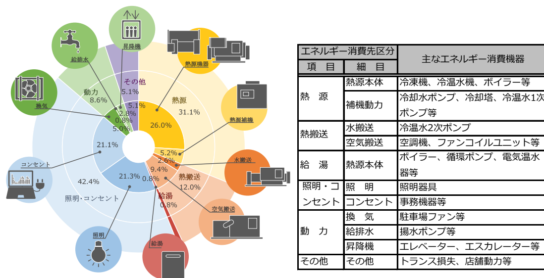
図 4-35 オフィスビルのエネルギー消費構造の例（中央熱源方式 34 のビル想定の場合）
