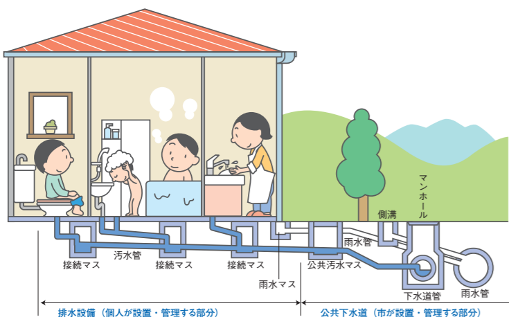
▲一般家庭の排水処理構造
