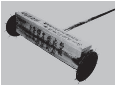
中枝式播種器
