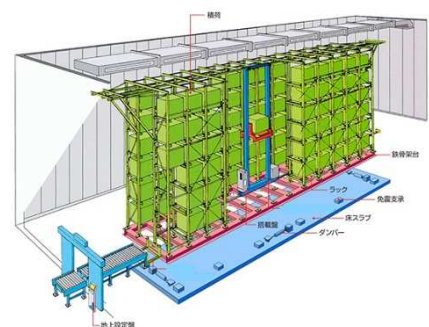
▲自動ラック倉庫免震システム
