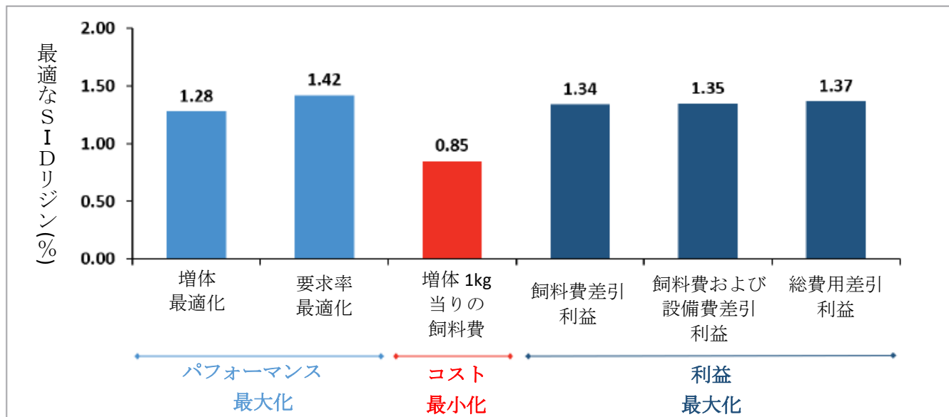
図 A2. PIC 豚(11.5~22.5kg の豚、PIC 社内部データ)に対し、それぞれの結果を最適化するための SID リジン値の例
