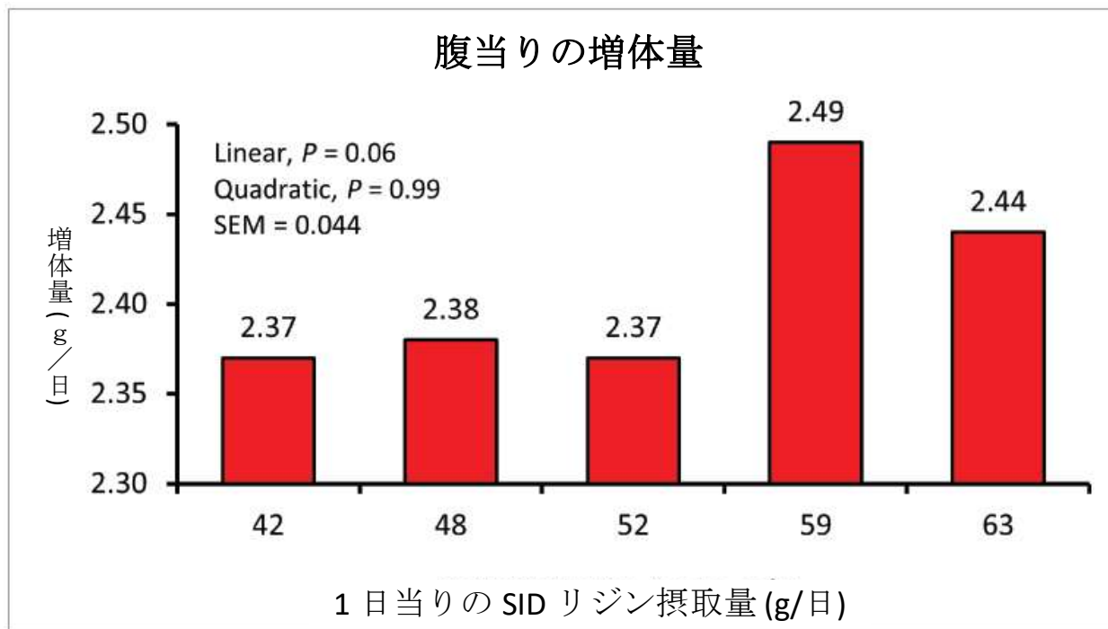
図 12. 授乳期の初産豚の腹当り増体量に対する SID リジンの 1 日当り摂取量の影響 (Bruder et al., 2018).
