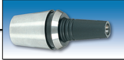
ER GTI (ER Collet with Tapping Holder)
