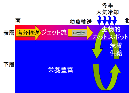
図2 ジェット流と生物的ホットスポットの形成メカニズム
