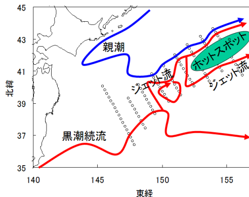
図1 北西太平洋における生物的ホットスポットとジェット流の分布。丸印は若鷹丸の調査点
