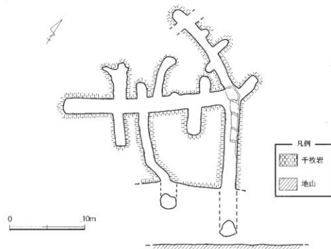
第4図 鉢山跡 平面図・壕口立面図
