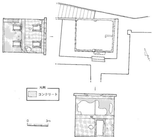
第16図 公益質屋跡平面図及び断面図
