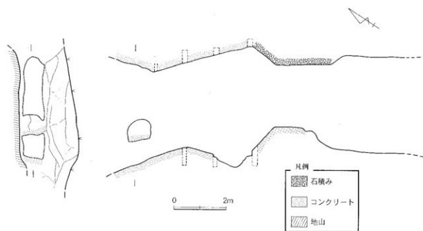
第18図 山グシの陣地壕平面図及び壕口立面図
