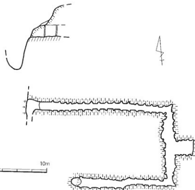
第10図 奉安壕平面図及び壕口断面図
