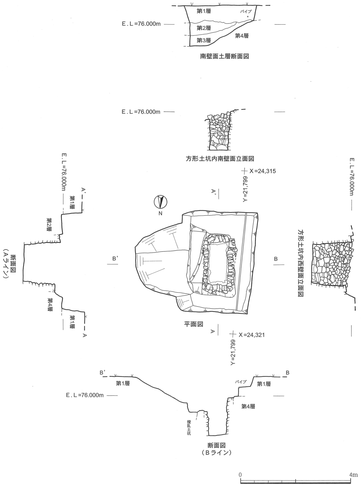
第4図 遺構平面図・断面図・立面図
