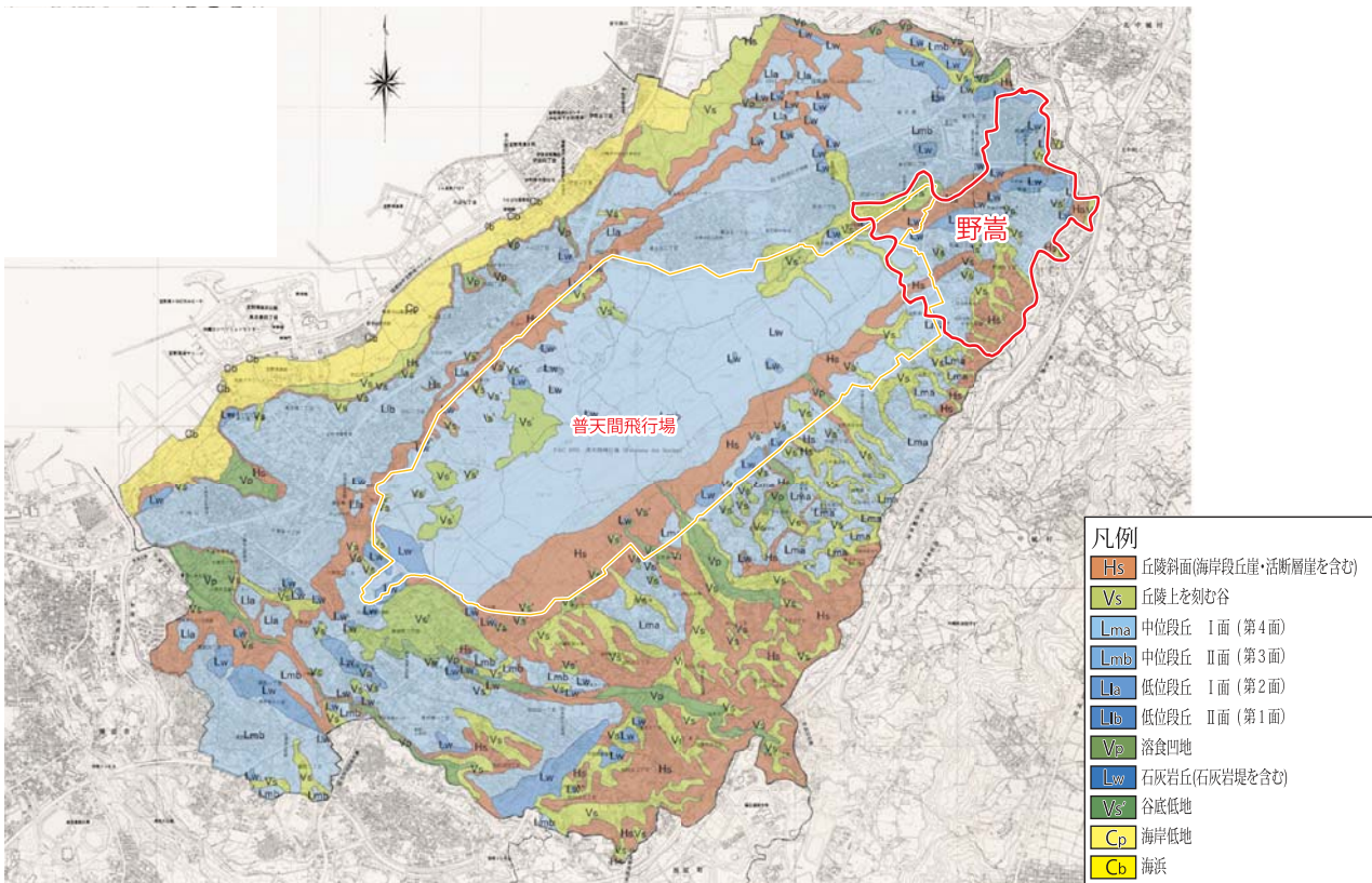
第Ⅱ-3 図 宜野湾市地形分類図
