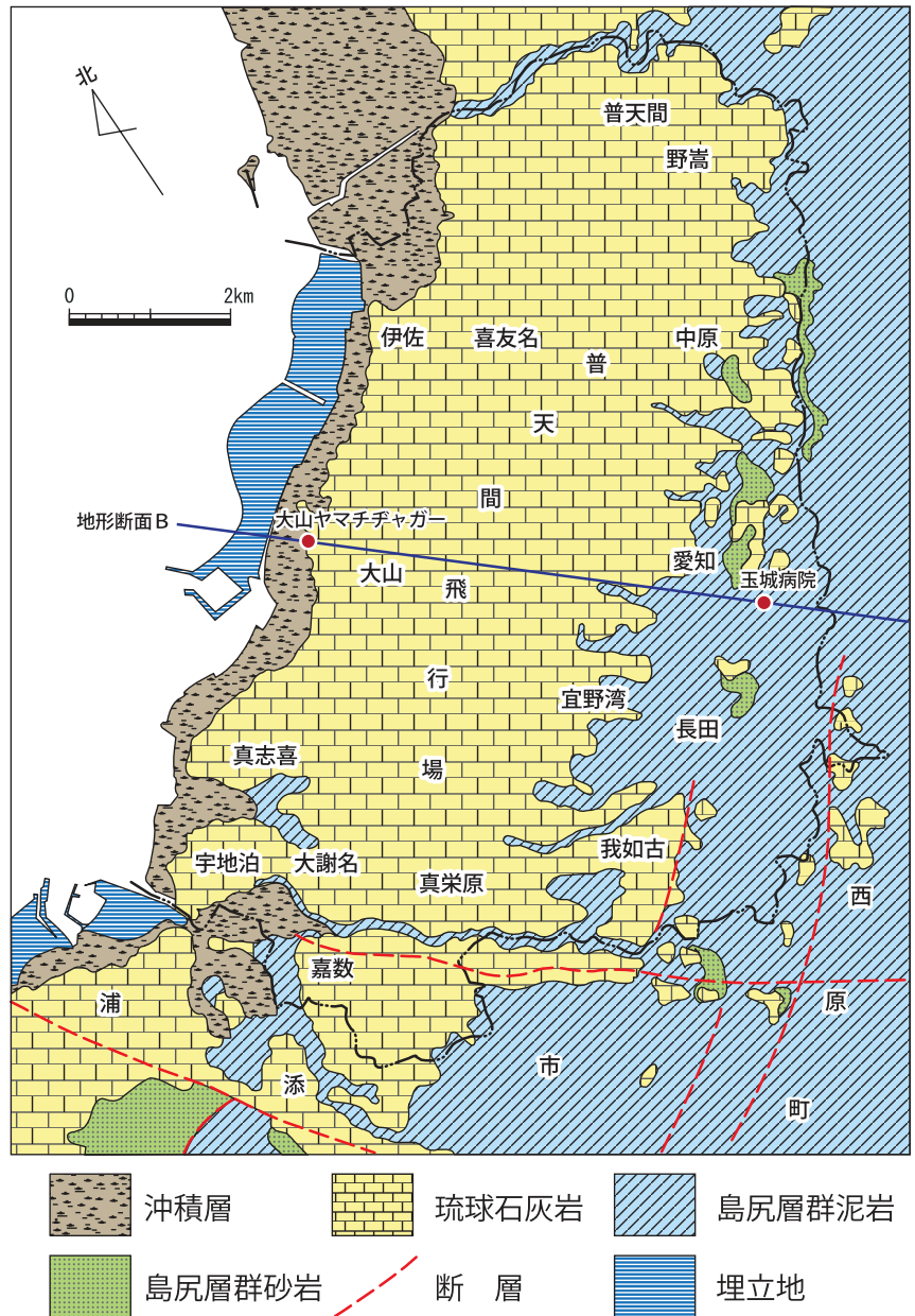
第Ⅱ-2図 宜野湾市の地質図
