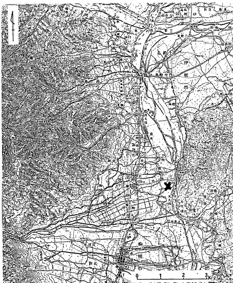
第1図 位置図
