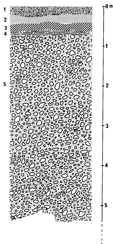
第5図 層序図
