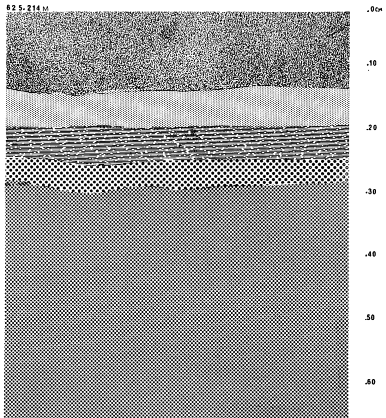
第2図 地層図
