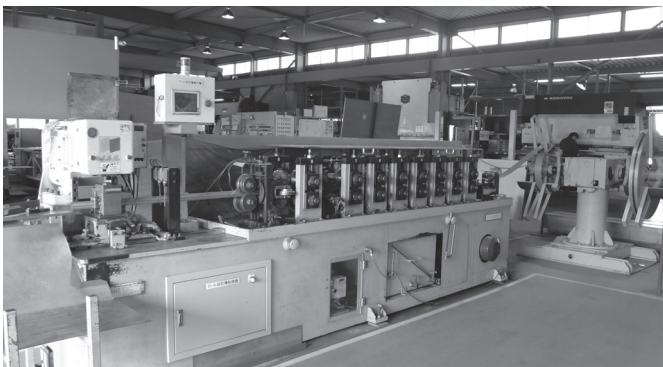
ロール成形ライン
