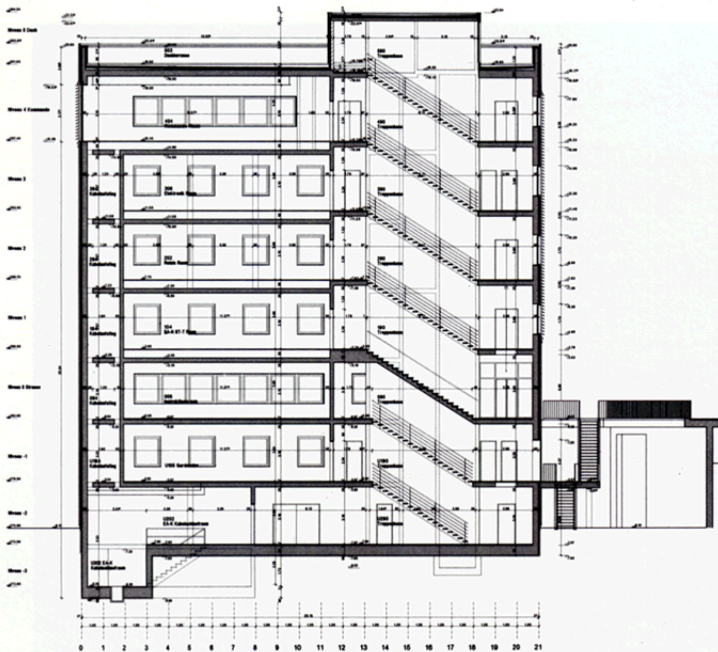
Section longitudinale / Longitudinal section
