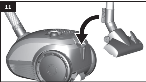
图 11 如果您需要暂停吸尘，可使用吸尘器侧面的辅助站立装置。 关闭电器后，将吸尘头上的钩子滑入吸尘器侧面的凹槽。
