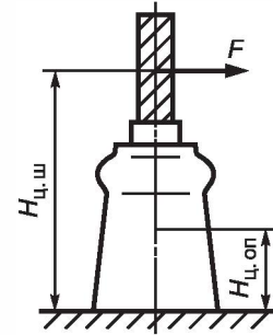
Рисунок 8 — К расчету приведенной массы опоры
