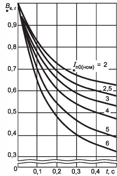
Рисунок 11 — Кривые для определения B_{*к.г} от синхронных генераторов с диодной бесщеточной системой самовозбуждения
