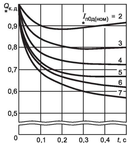
Рисунок 16 — Кривые для определения Q_{*к.д} от синхронного электродвигателя
