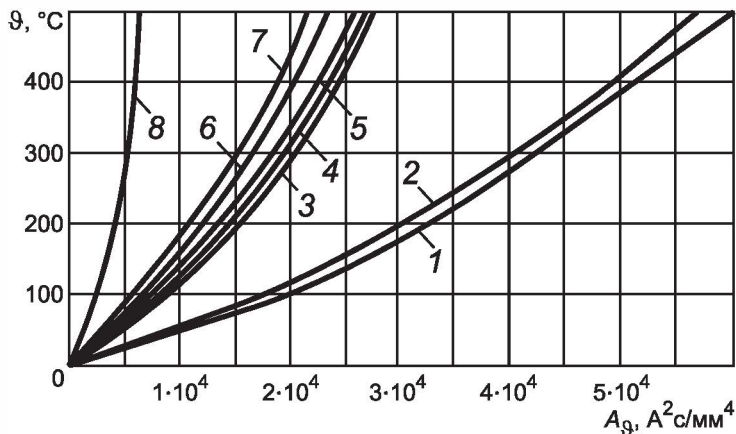
Материалы проводников: 1 — ММ; 2 — МТ; 3 — АМ; 4 — АТ; 5 — АДО, АСТ; 6 — АДЗ1Т1; 7 — АДЗ1Т; 8 — СтЗ
