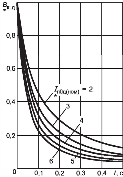
Рисунок 17 — Кривые для определения B_{*к.д} от асинхронного электродвигателя
