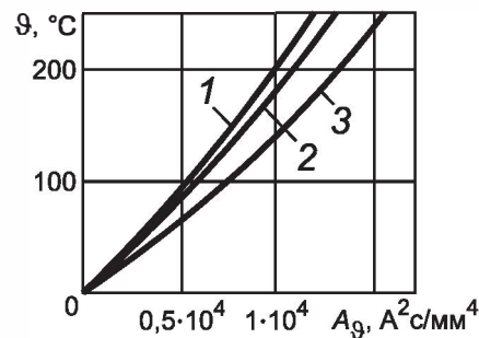
Материалы проводов: 1 — сплавы АЖ и АЖКП; 2 — сплавы АН и АНКП; 3 — алюминий марок А, АКП, АпКП и сталеалюминий марок АС, АСКП, АСКС, АСК, АпС, АпСКС, АпСК
