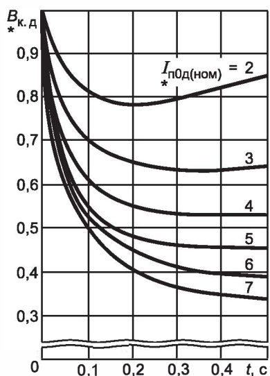
Рисунок 15 — Кривые для определения B_{*к.д} от синхронного электродвигателя
