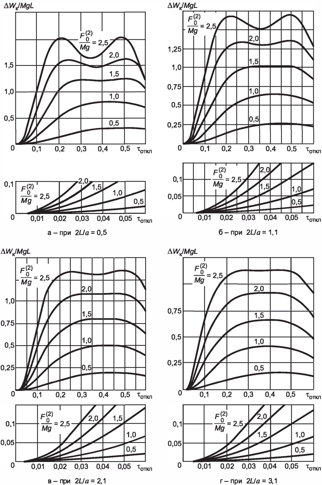
Рисунок В.2 — Зависимость \Delta W_{\kappa}/(MgL) от относительной продолжительности двухфазного КЗ
