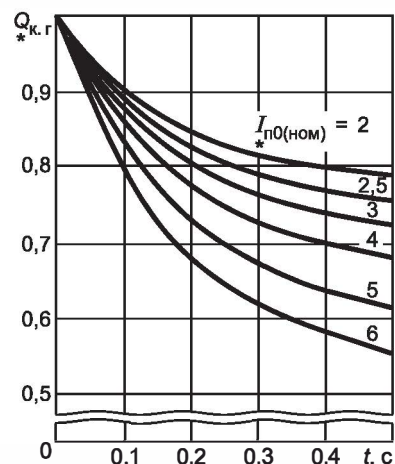
Рисунок 14 — Кривые для определения Q_{*к.г} от синхронных генераторов с диодной бесщеточной системой самовозбуждения
