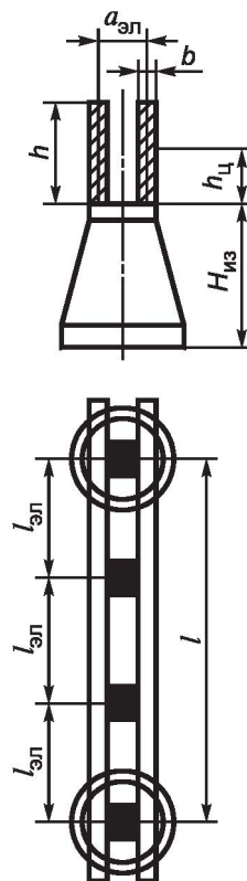
Рисунок 4 — Двухполосная шина
