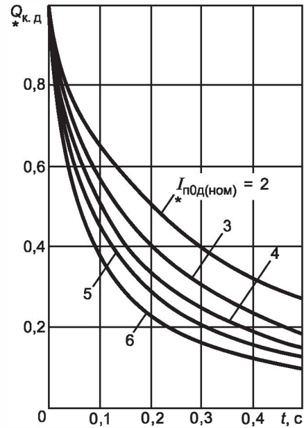
Рисунок 18 — Кривые для определения Q_{*к.д} от асинхронного электродвигателя
