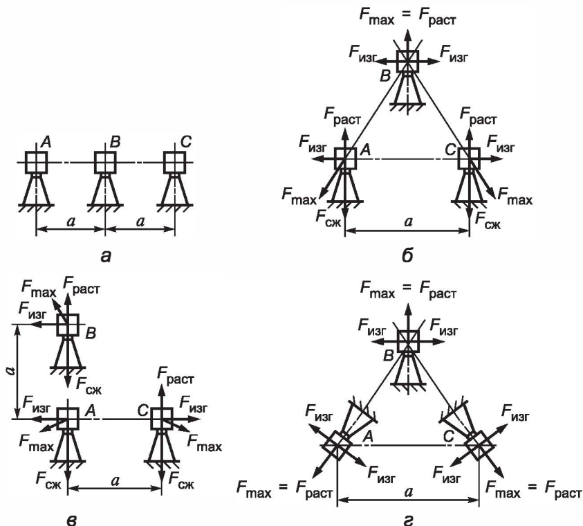
Рисунок 2 — Схемы взаимного расположения шинных конструкций
