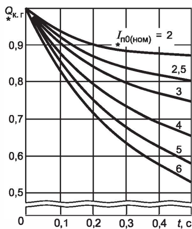
Рисунок 13 — Кривые для определения Q_{*к.г} от синхронных генераторов с тиристорной системой самовозбуждения
