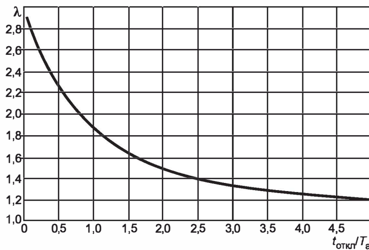
Рисунок В.1 — Зависимость коэффициента \lambda от t_{\text{откл}}/T_a
