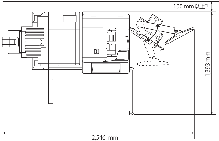
中綴じフィニッシャー・F1+ マルチカラーイメージリーダーユニット装着時
