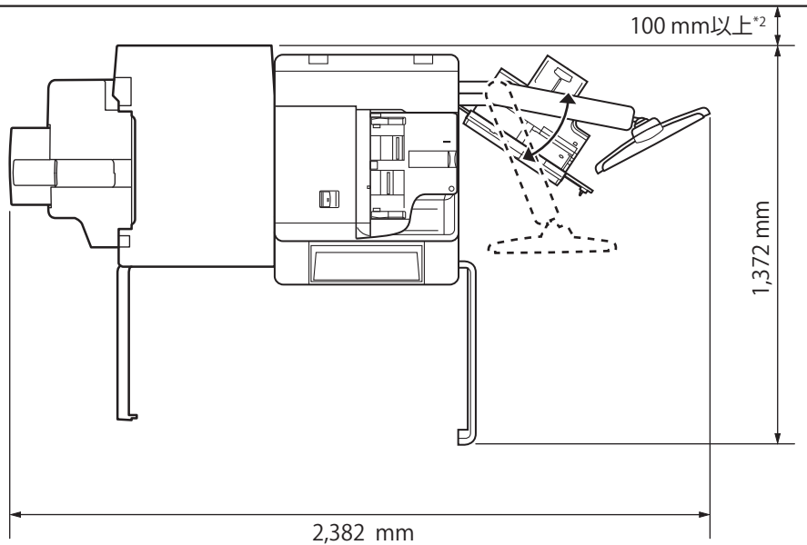
中綴じフィニッシャー・D1+ マルチカラーイメージリーダーユニット装着時
