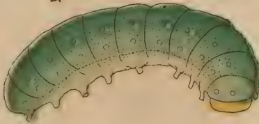
Fig. 89.—Sesame caterpillar.
