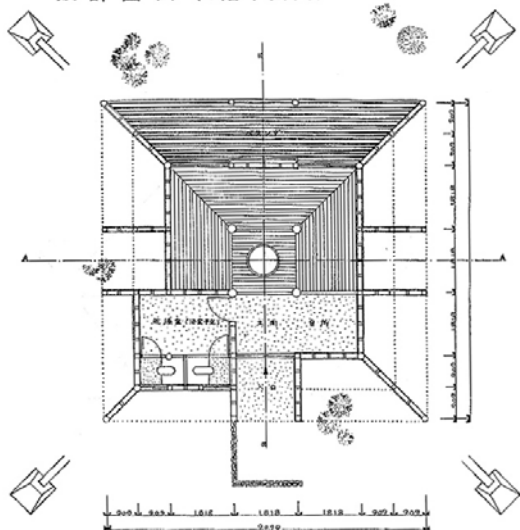
設計図面 (1階平面図)
