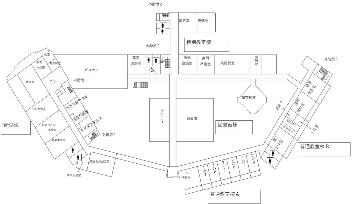
1階平面図
