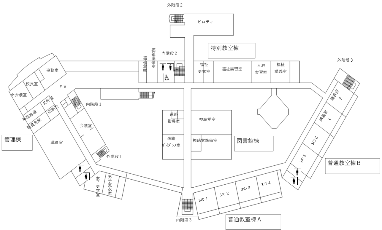
2階平面図
