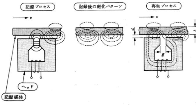
交流バイアス法 (東北大 永井健三)
