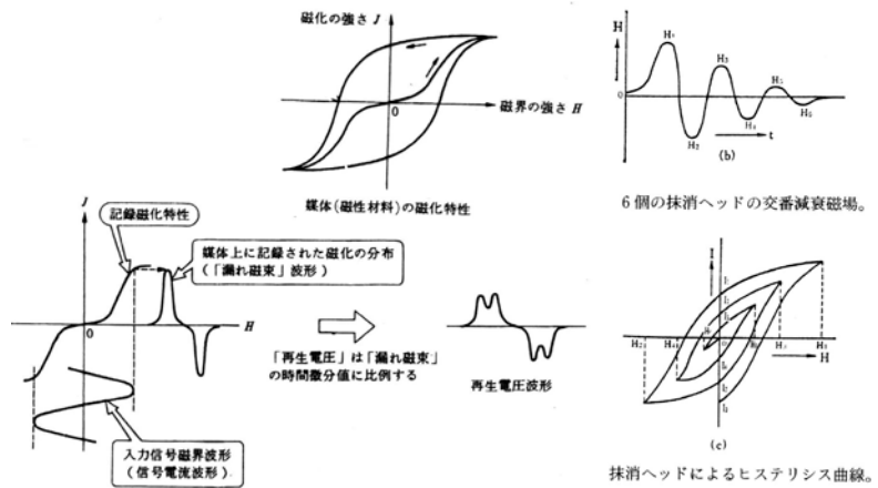
交流バイアス法 (東北大 永井健三)
