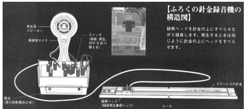
ポールセンの磁気記録 (1898) (針金録音機 学研)
