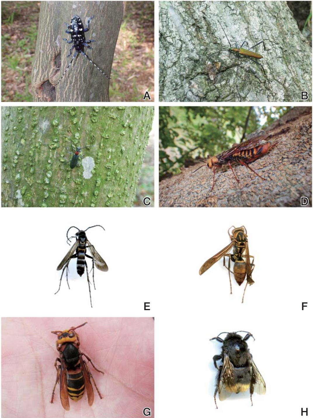
図6 宍道湖グリーンパークの昆虫類(3).
