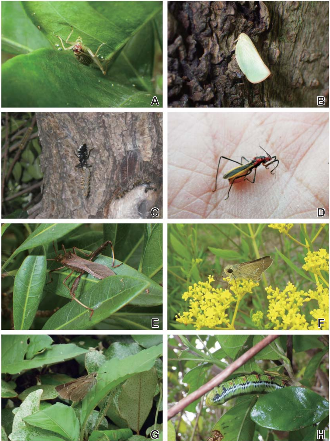
図4 宍道湖グリーンパークの昆虫類(2).
