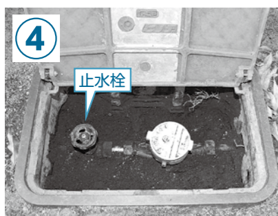
水道メーター器ボックス内の止水栓 (右に回すと水が止まる)
