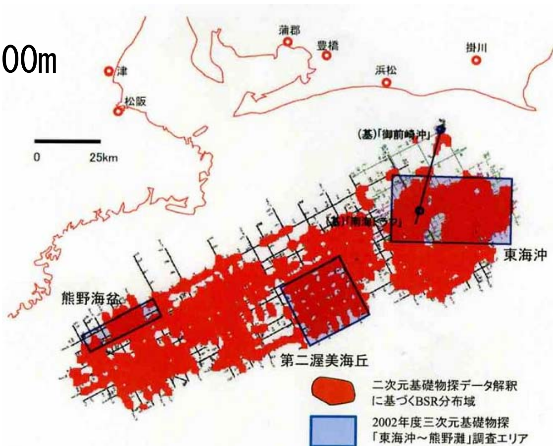
南海トラフでのBSR分布
