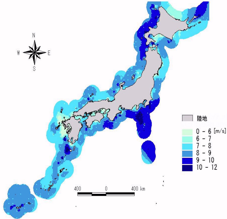
沿岸域100kmの年平均風速(60m高)
