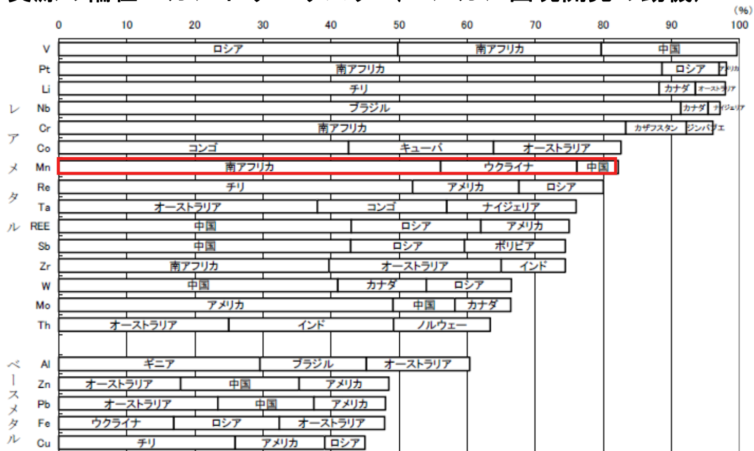
図 2.3. レアメタルとベースメタルの国別埋蔵シェア（上位 3 カ国）
