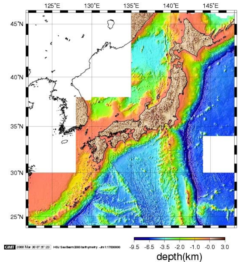
日本近海の水深分布
