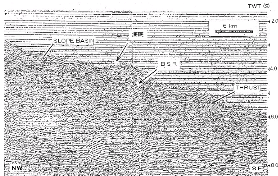
海底擬似反射面 (BSR) 日本バルカー HP
