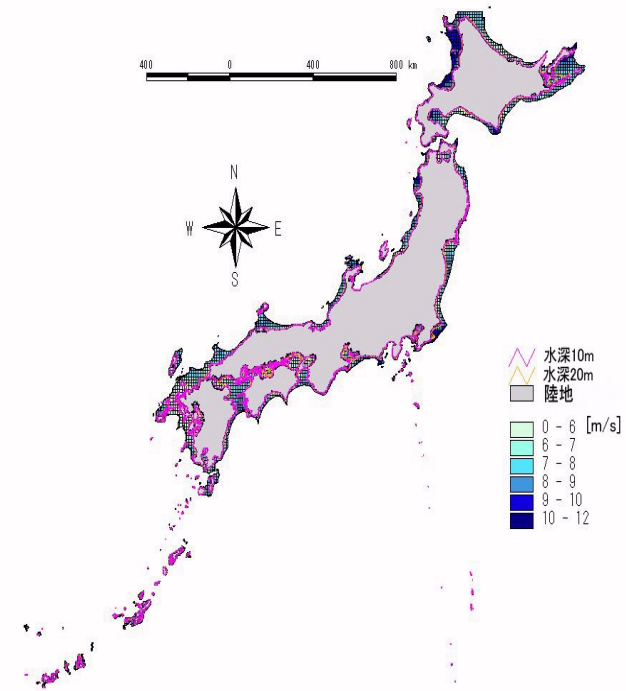
水深100m未満の風速分布(60m高)
