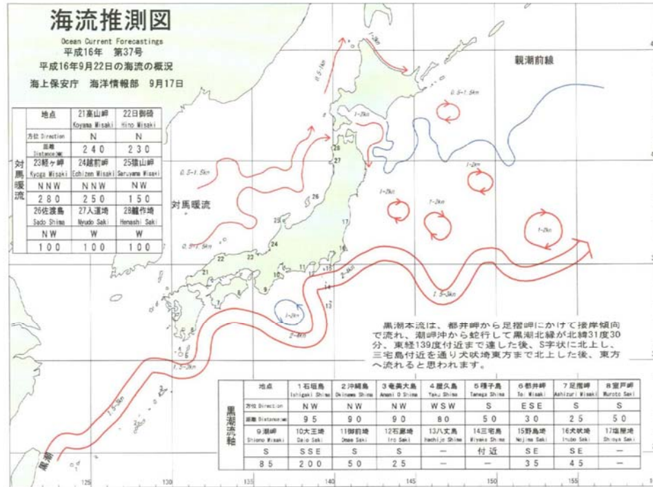
2004年9月22日の海流推測図
