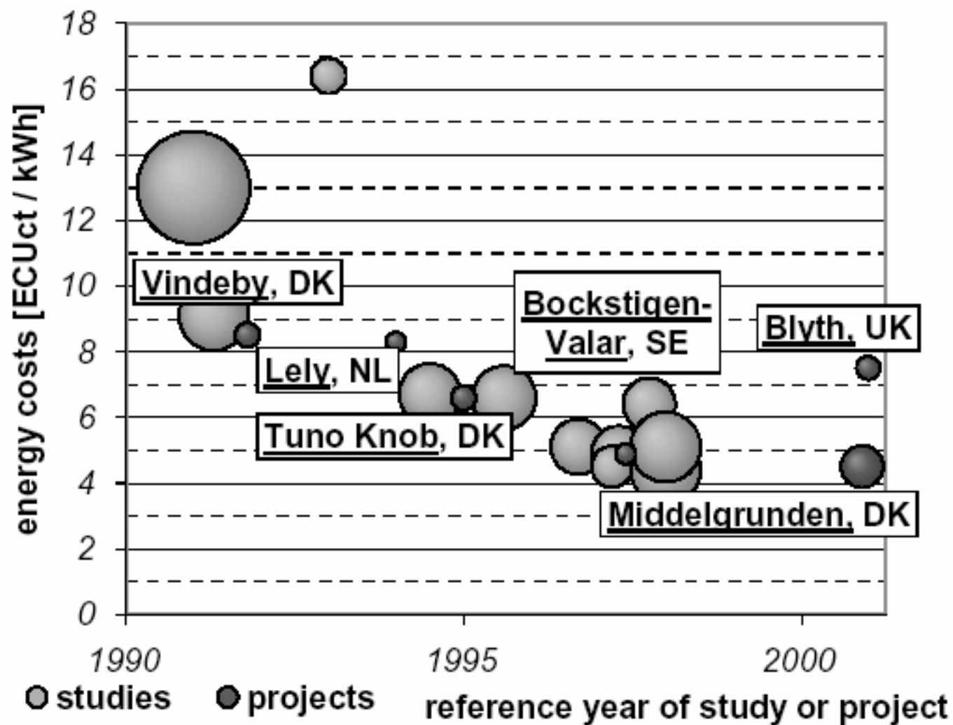
Fig. 4: Reduction in Cost (Kühn et al, 1998) (Sørensen et al 2000)
