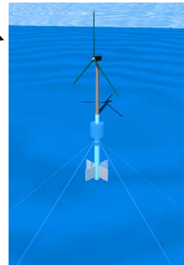
スパー型 (円筒型) ＜沿岸外洋＞
