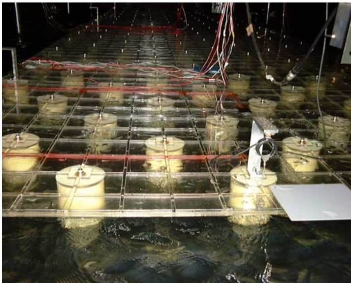
水槽実験
