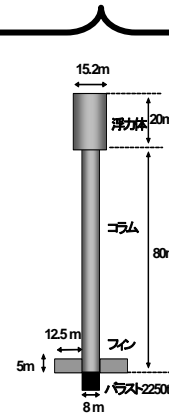
Dコラム80m
