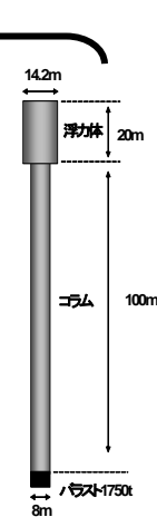
Gコラム100m
